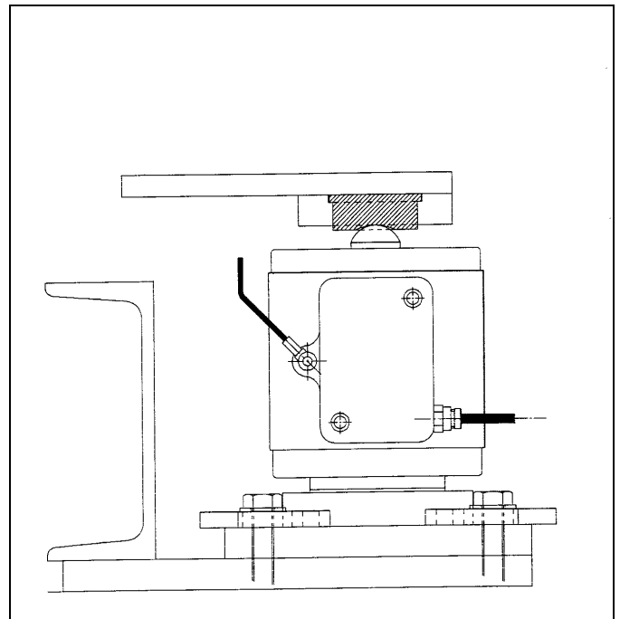
Montage sur récepteurs de charge variantes B et C
