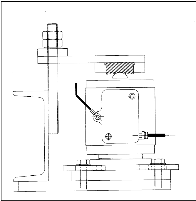
Montage sur récepteur de charge variante A transportable sans démontage
