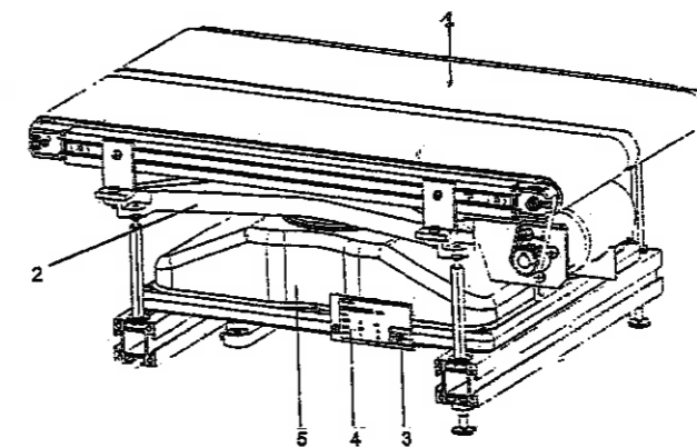
Vue E - Récepteur de charge type 10A
