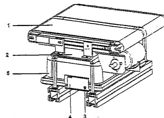
Vue E - Récepteur de charge type 10B
