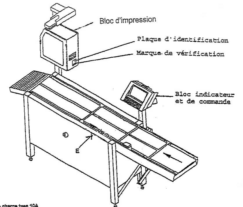
Vue E - Récepteur de charge type 10A
