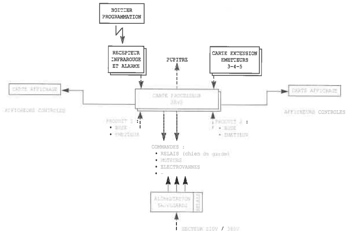
Double face 5 produits
