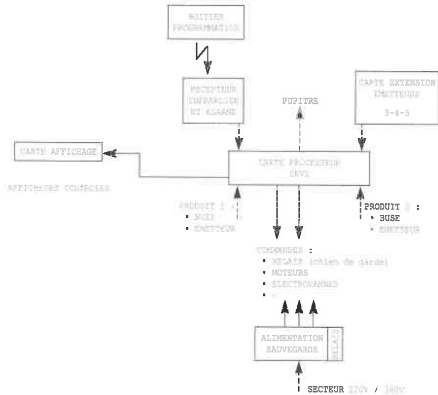
Schéma synoptique simple face 5 produits
